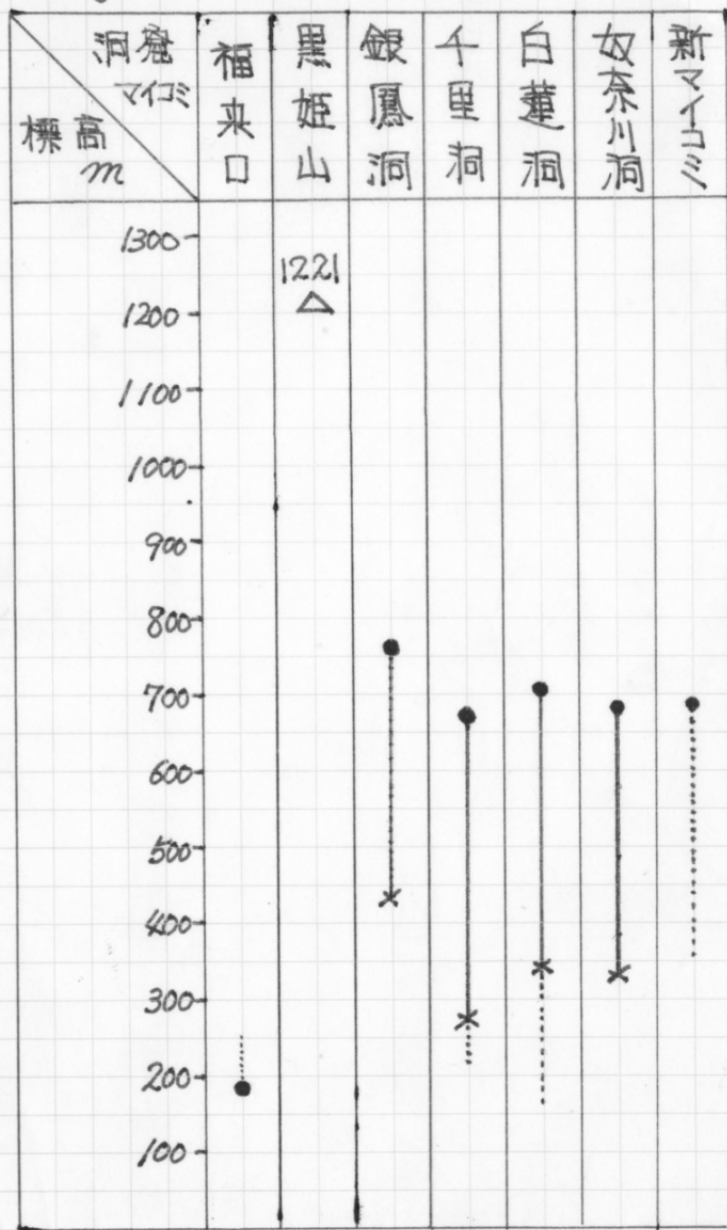
Fig-1 マイコミ平の水準の比較
