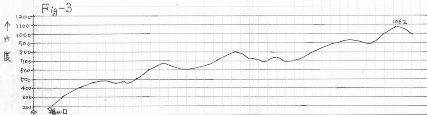
福加口よりマイコミ平の南の水準点1062への断面図(ちょうどこの線は田海川の沢づたいを走っている) 2万5千分の1で高さも横と同縮尺である。
